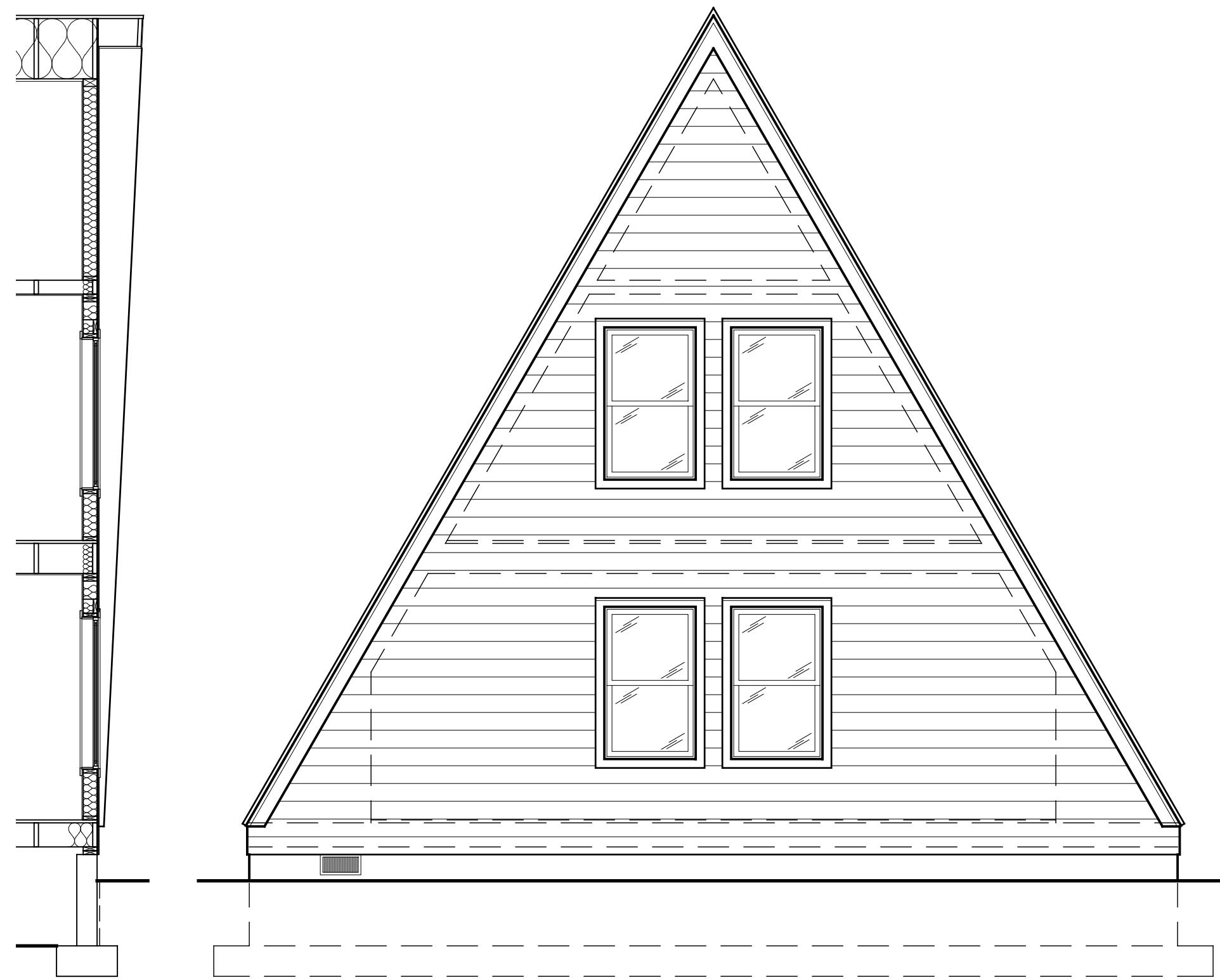
ELEVATION
